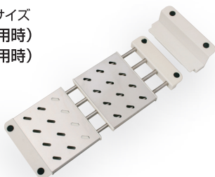
TDG-43 砥石用スライドラック サイズ 約2950×137×55mm 標準小売価格 1,650円 入数10 4966684060203
